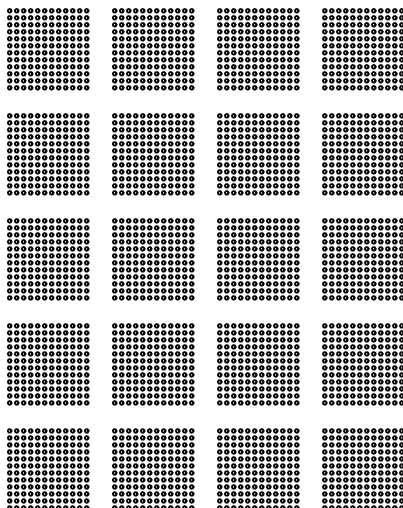
Chess fältperforering \varnothing 5 mm. Kvadratisk delning 10 mm. Fri area 12,5%.
