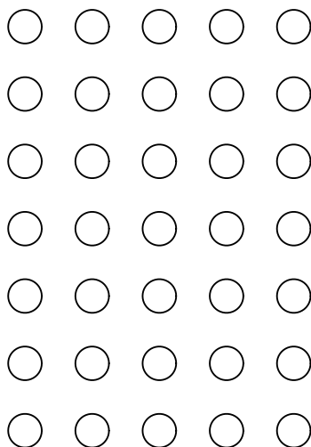
Perforering \varnothing 5 mm. Kvadratisk delning 10 mm. Fri area 20%.
