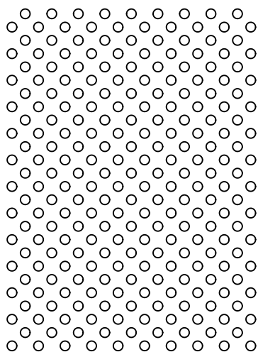
Perforering \varnothing 1,8 mm. Kvadratisk diagonal delning 3,5 mm. Fri area 21%.
