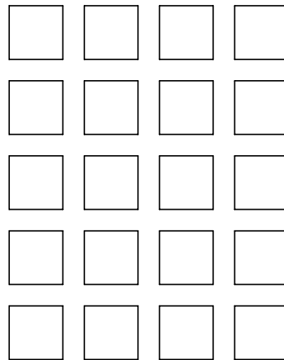
Fyrkantperforering 10x10 mm. Kvadratisk delning 14 mm. Fri area 51%.
