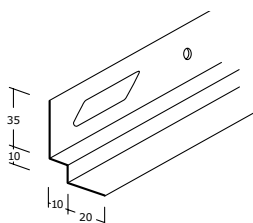
Skuggprofil med nabb 8858
