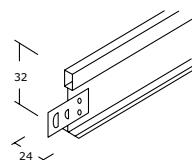
Tvärprofil
