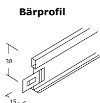
Bärprofil
