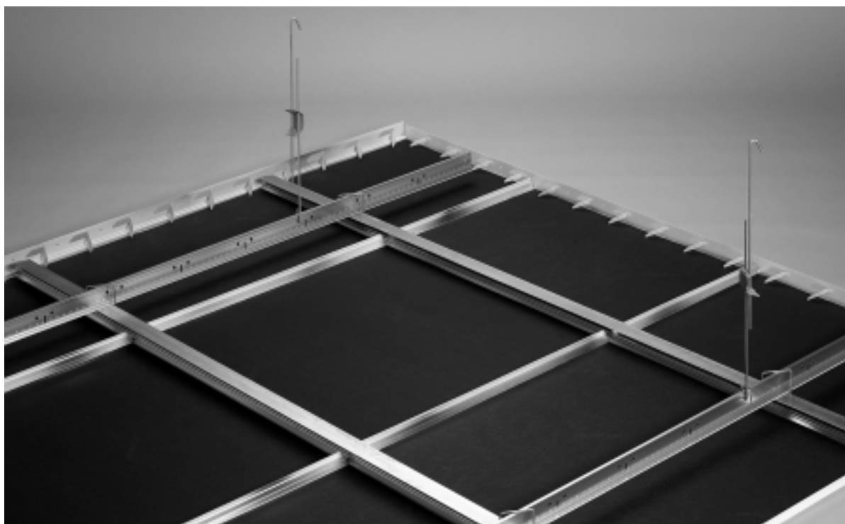
Pendelfäste 8854
