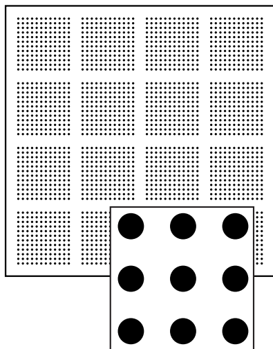
Chess fältperforering 5 mm, kvadratisk delning 10 mm. Fri area 12,5%.
