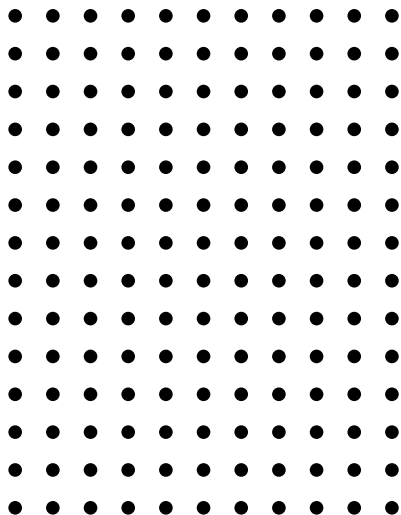
Perforering 1,8 mm, kvadratisk delning 5 mm. Fri area 10,3%.
