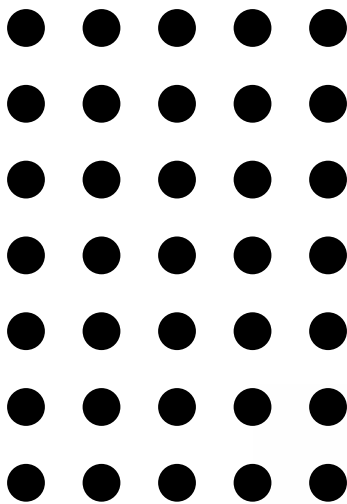
Perforering 5 mm, kvadratisk delning 10 mm. Fri area 20%.
