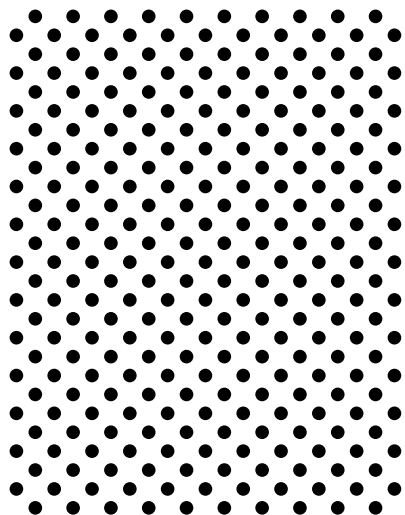
Perforering 1,8 mm, kvadratisk diagonal delning 3,5 mm. Fri area 21%.
