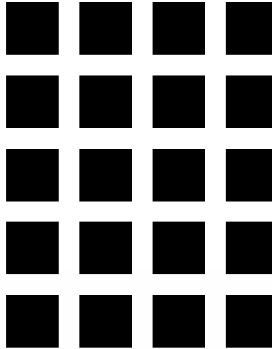
Fyrkantperforering 10 mm, kvadratisk delning 14 mm. Fri area 51%.
