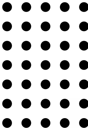
Perforering Ø5 mm. Kvadratisk delning 10 mm. Fri area 20%.
