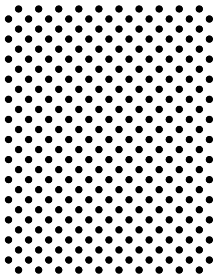
Perforering Ø1,8 mm. Kvadratisk diagonal delning 3,5 mm. Fri area 21%.
