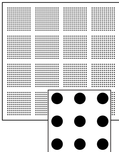
Chess fältperforering Ø5 mm. Kvadratisk delning 10 mm. Fri area 12,5%.
