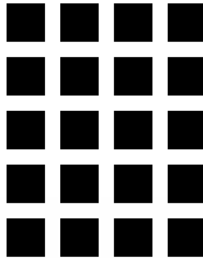
Fyrkantsperforering 10 mm. Kvadratisk delning 14 mm. Fri area 51%.
