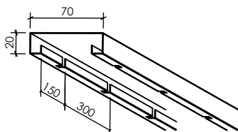
Hakprofil U (9676) Längd: 2400
