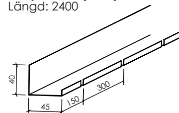
Hakprofil VU (9670) Längd: 2400
