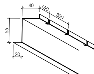
Hakprofil VU (9670) Längd: 2400
