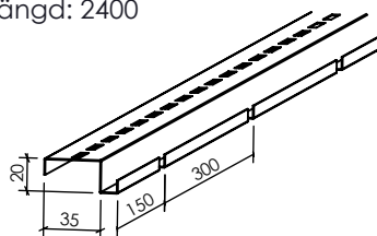
Hakprofil V (9679) Längd: 2400
