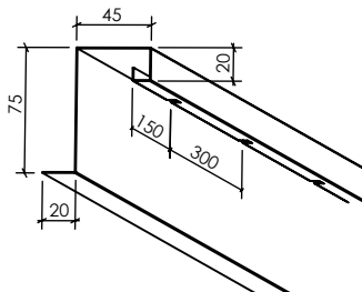
Hakprofil V (9679) Längd: 2400
