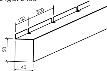
Hakprofil K (9667) Längd: 2400
